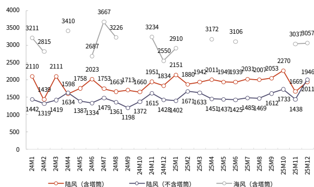
图 4：2024 年起国内风电机组月度中标均价
