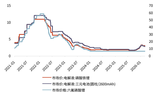
图 10: 电解液、六氟磷酸锂 (右轴) 价格 (截至 2026/3/6)
