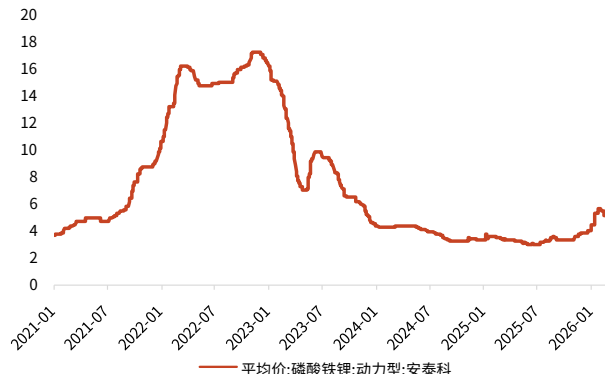
图 8: 动力型磷酸铁锂价格 (截至 2026/3/6)
