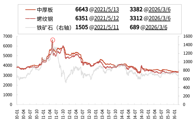
图 5：国内中厚板、螺纹钢、铁矿石价格（截至 2026/3/6）
